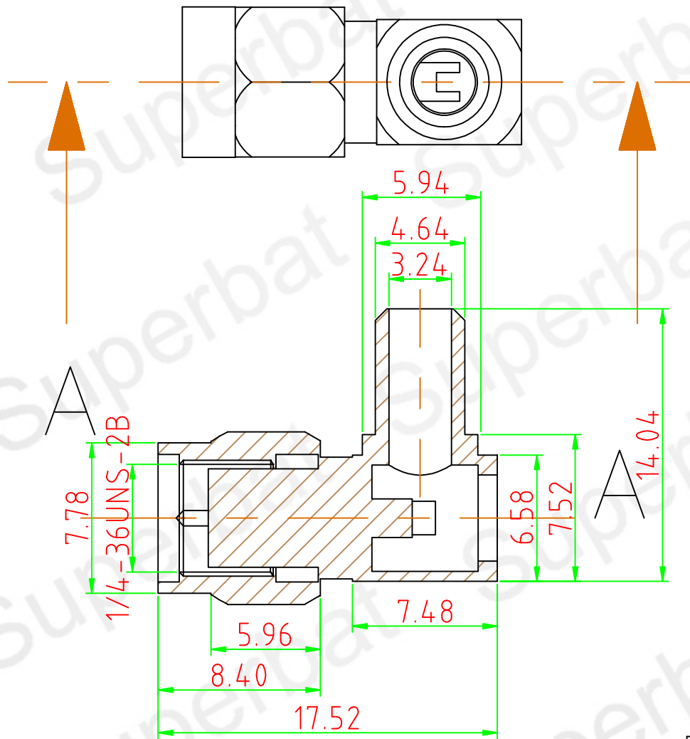
SECTION A-A
